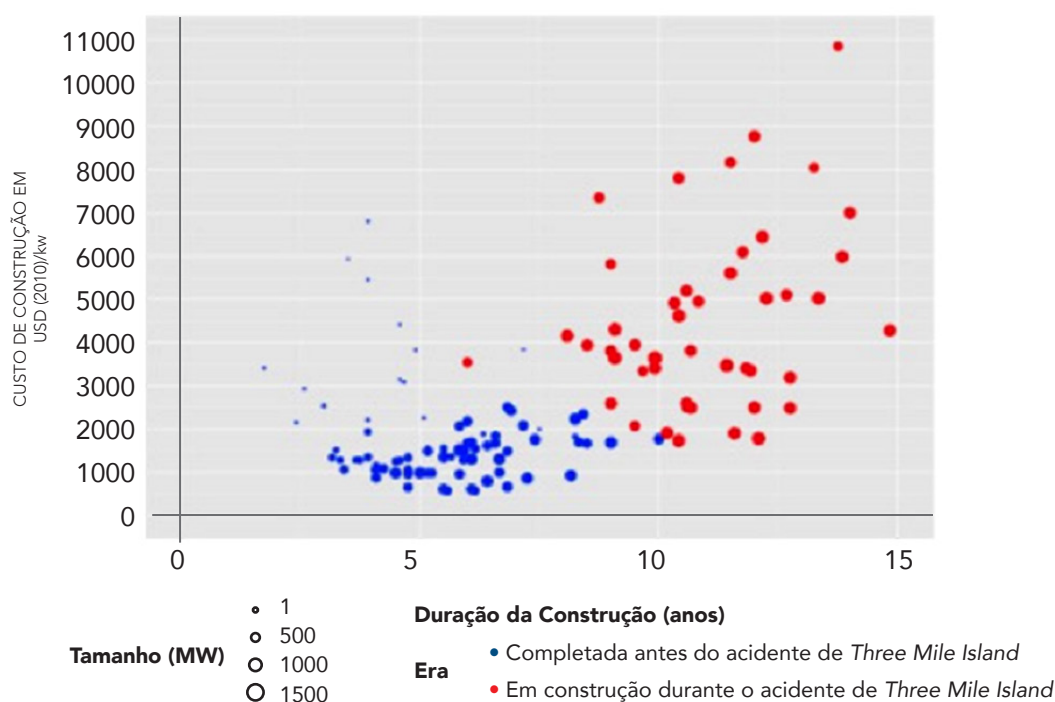
Figura 2: Custo (overnight) e duração da construção de usinas nucleares dos EUA. 13
